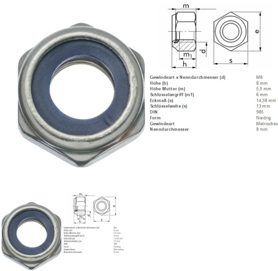
Sechskantmutter M8-A2-70 ISO 7040 Selbstsichernd
