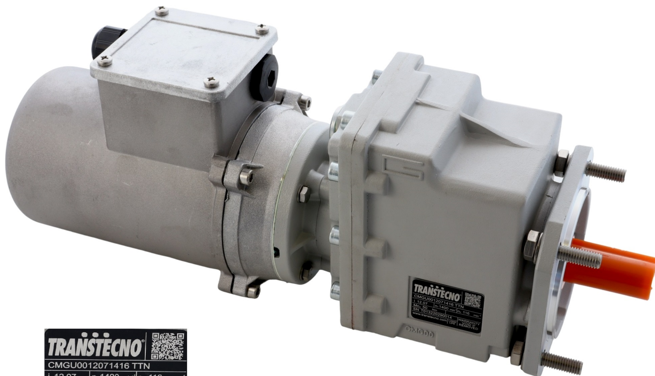
Rawa Motor für Istobal 0,25KW 230/400 V 50HZ 116UPM
