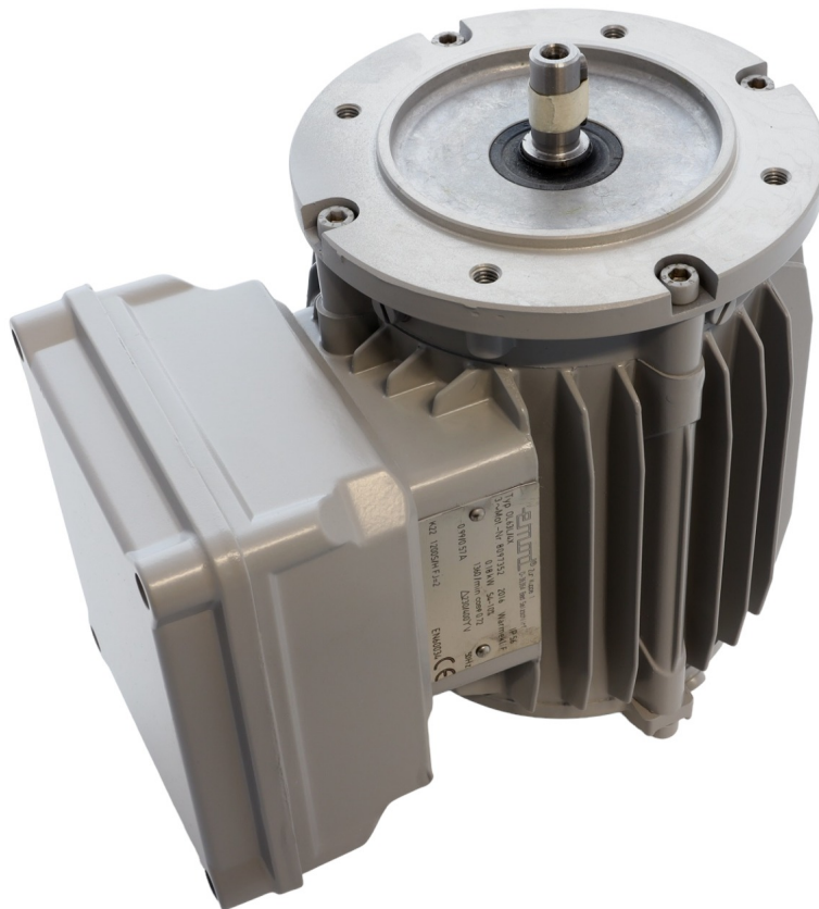
Motor für Nufa 6-1677 SB Verfahrantr. links 0,18 KW 63/4
