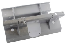
Laufwagen WS SB Links 251251 Verzink und Lackiert für Waschstraße SL 2
