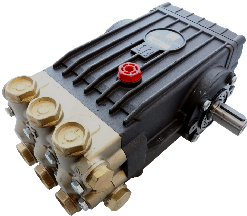
HD-PUMPE Interpump WS102 21 L/MIN 100 BAR 1450U/min-4,0KW Serie 47
