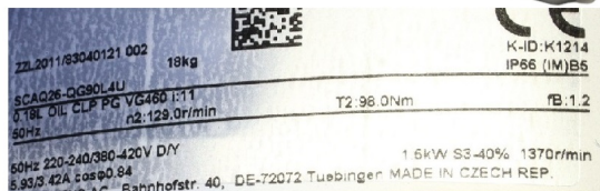
Getriebemotor Siemens / Inomotics 1,5KW 230/400V50HZ I=11/ 129 UPM Dachbürstenrotation Nufa 6-395+Maxi Vario
