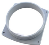
LAGERFLANSCH FÜR METALLRING GEHÄUSESEITE für Dachdüse Modular
