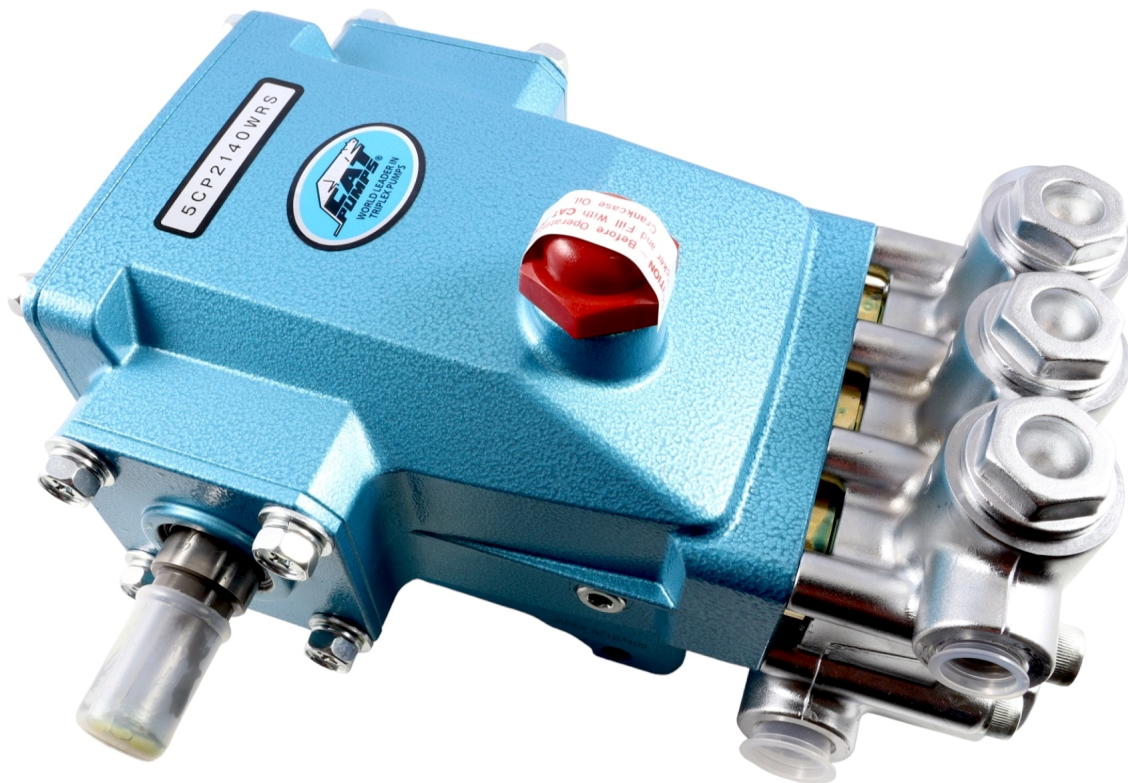
Cat Pumpe 5CP2140WF / 5CP2140WRS, 175 bar, 13 l/min, 1420 U/min, 4,7 kW, Antriebswelle links
