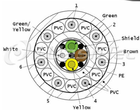
CAN-BUS LEITUNG Meterware (2X0,5+2X1,0)C+7X1,0
