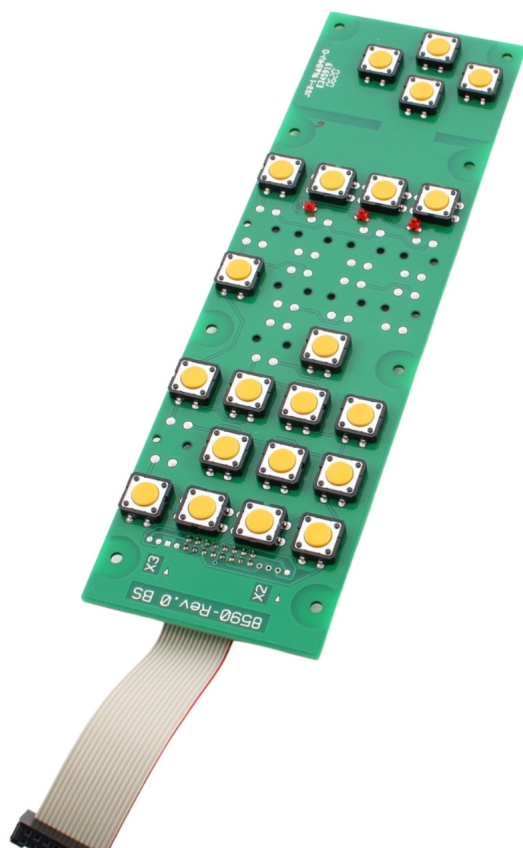
Bauteileträger Tastatur für Bedienterminal CP0-TASTATUR
