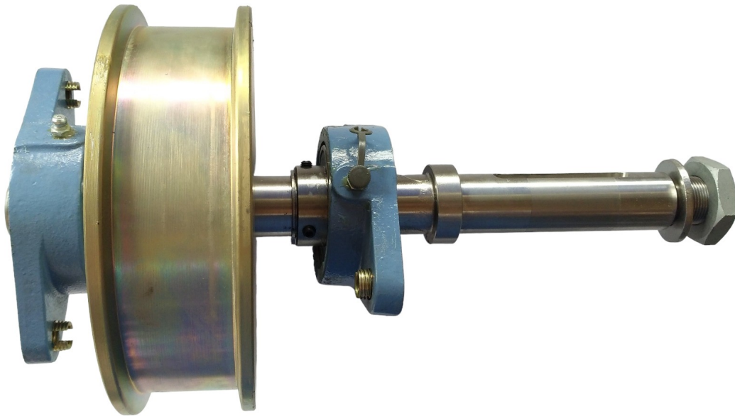
Antriebsrolle komplett mit Welle und Lager VMG Maxi Wash Pro Typ 6-0705
